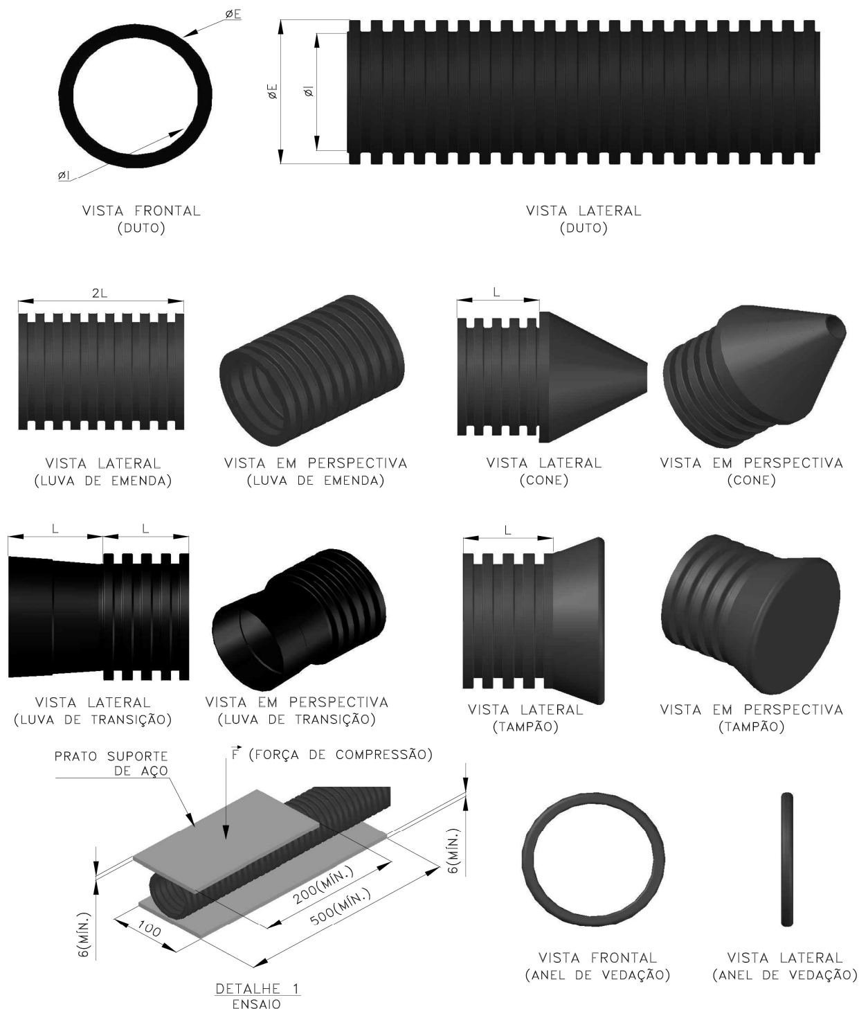
Figura 1 - Dutos Corrugados e Conexões
